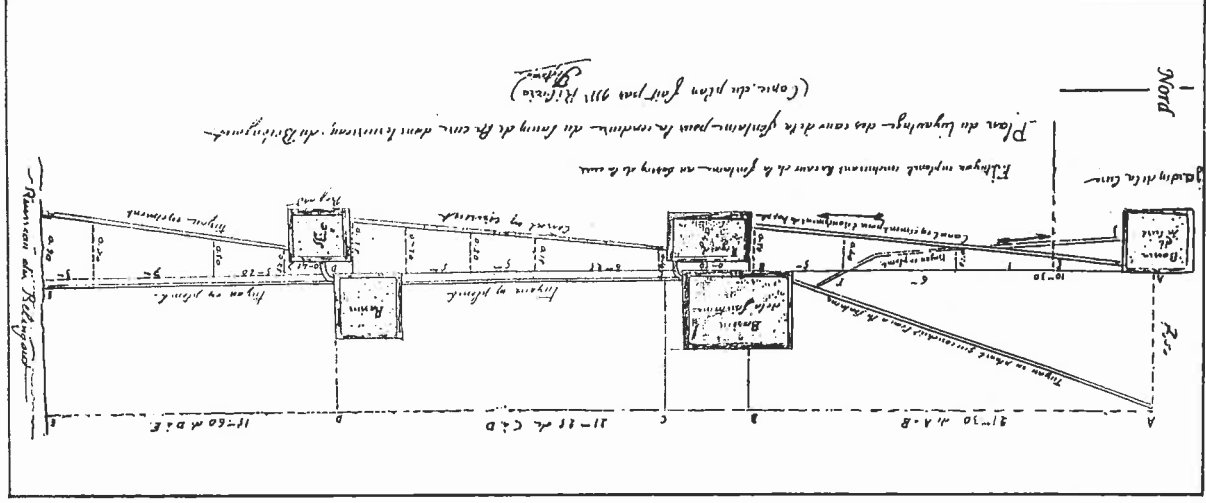
Fig. 3 - Plan des bassins, tuyaux, canaux et regards du jardin de l'abbaye, d'après le plan de M. Ribière (copie Peytavie, début du XX e s.). Les eaux arrivent de Griffoul en A (en haut et à gauche du plan) et gagnent le Bélingou (à droite du plan).
